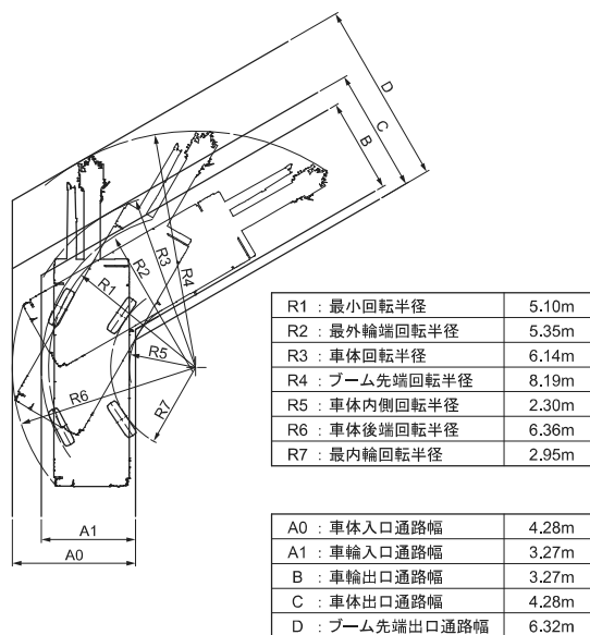
4輪ステアリングで右折する場合
