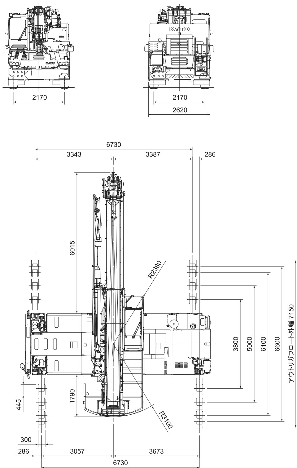
X型アウトリガ
